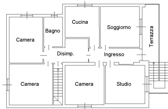
PIANTA PIANO PRIMO H=2,75
